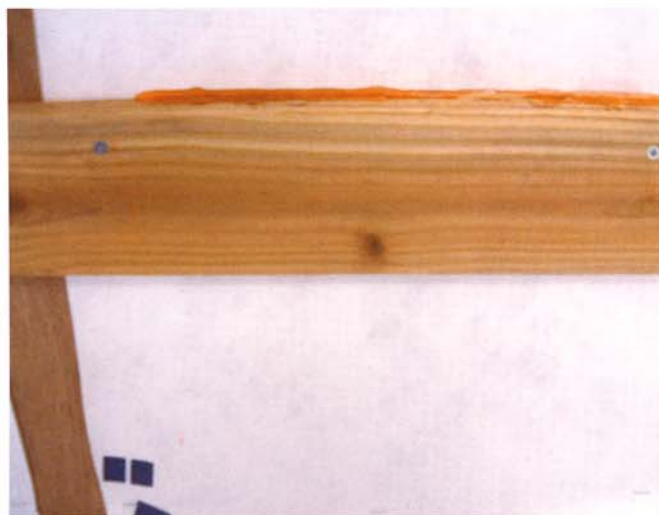
胴縁に水が溜まり、浸水の原因になる恐れがあります。
